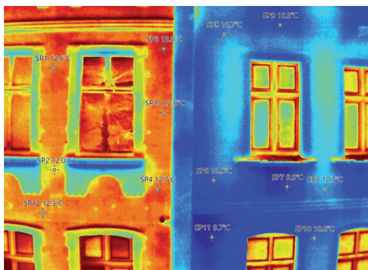
Porównanie innowacyjnej cienkowarstwowej powłoki termoizolacyjnej marki ECOBAUTER o grubości 1 mm z tradycyjnym systemem ocieplenia o grubości 15 cm
