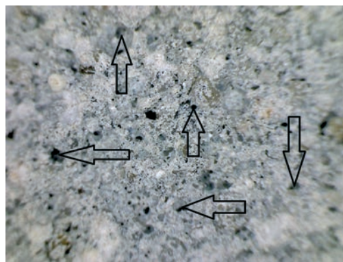
Tynk renowacyjny THERMOPAL SR 24 z widocznymi komorami powietrznymi (powiększenie x 200).
